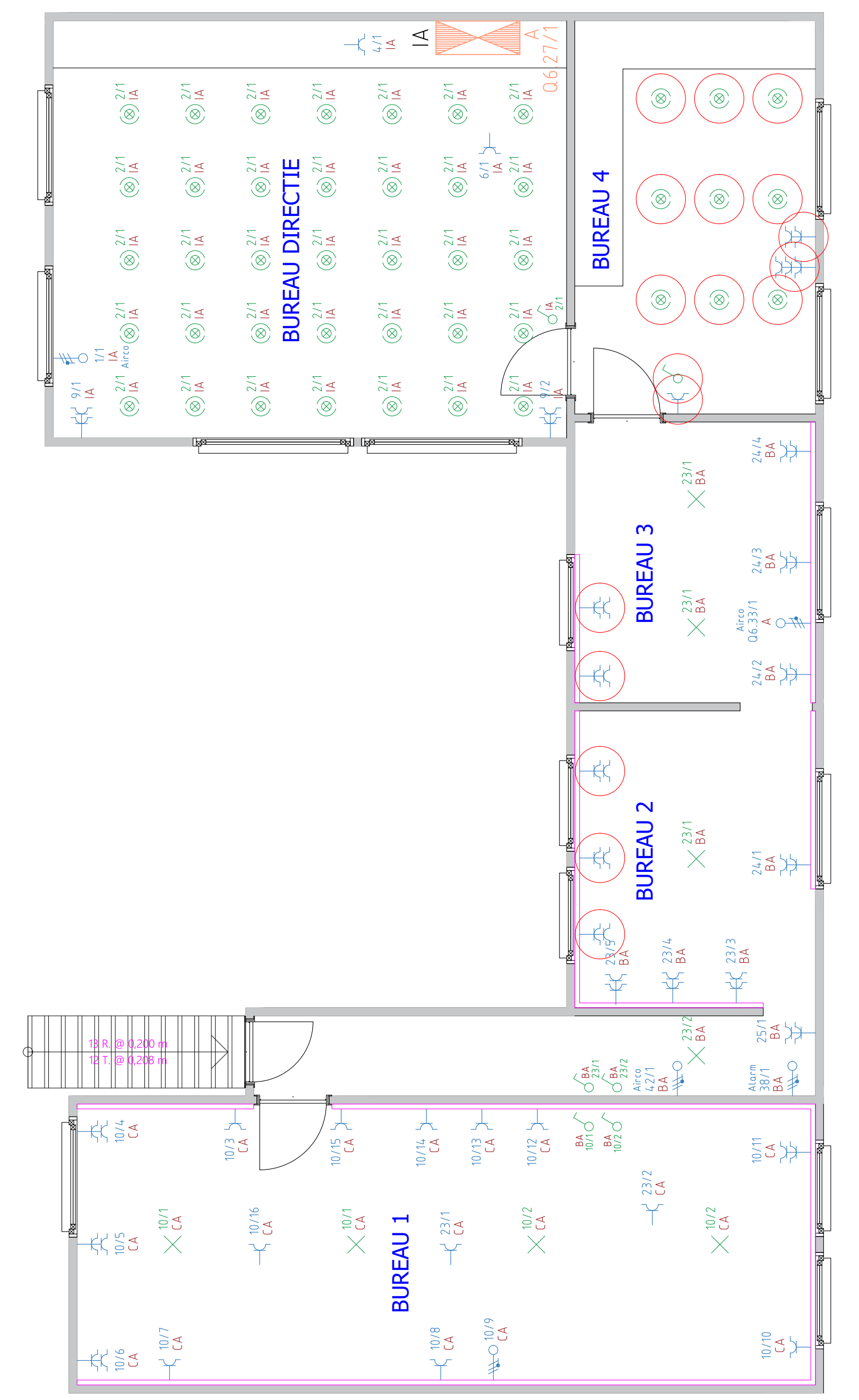
Verdiep bureaus 1/50
